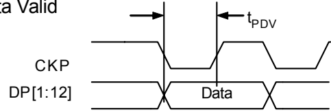
Data Valid
