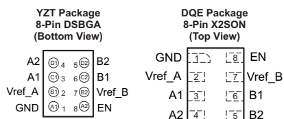
LSF0102
