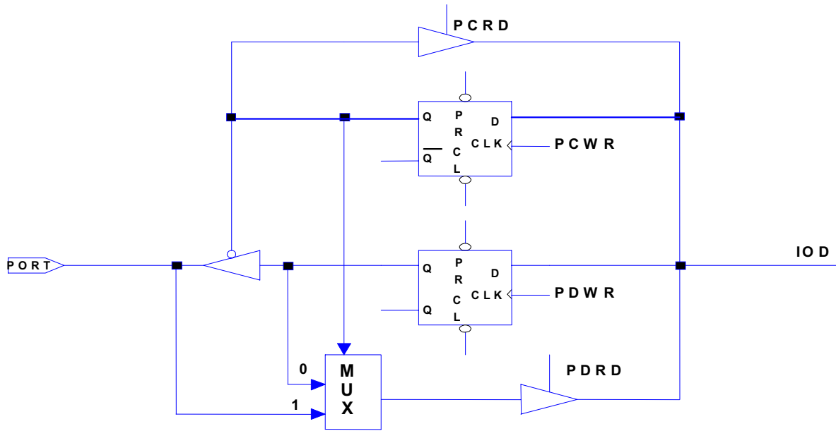
图 7 (a) I/O 端口电路和 I/O 控制寄存器
