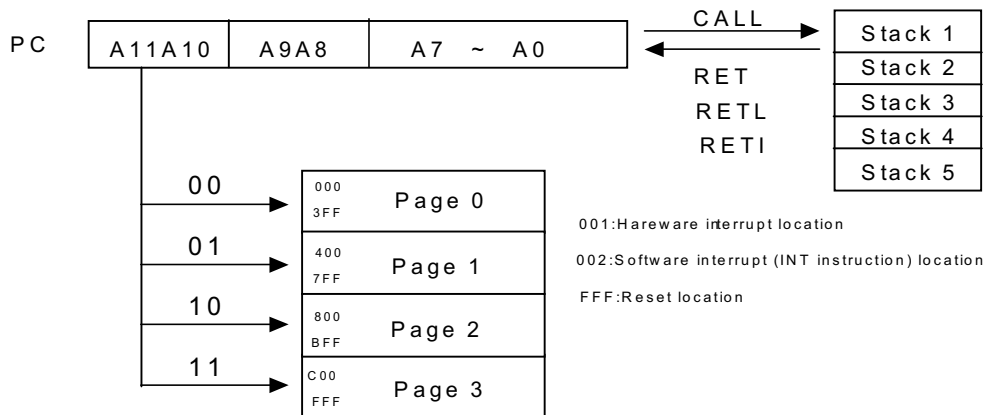
图 3 程序计数器结构
