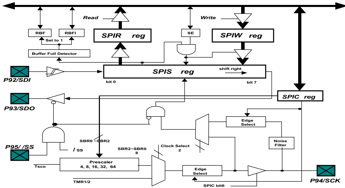
图 11 SPI 框图
