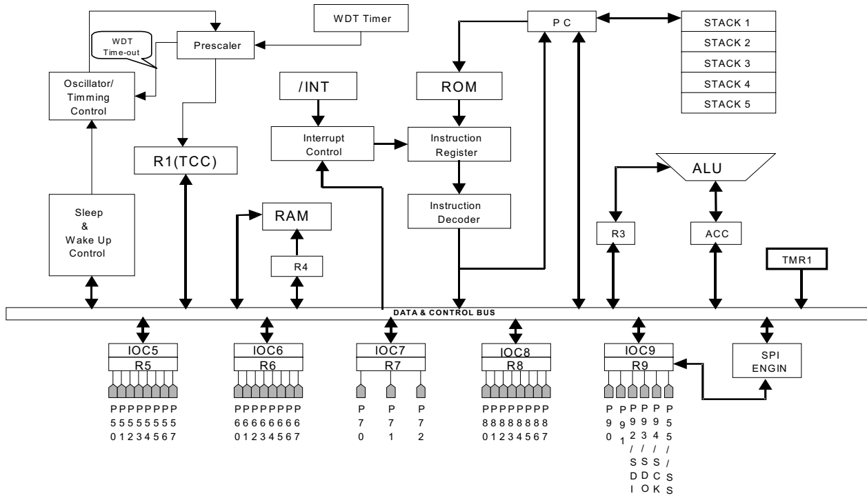
图 2 功能模块图
