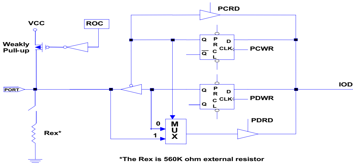
图 7(b)带 R-OPTION I/O 端口电路
