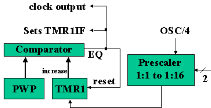
图 15 TIMER1 的框图
