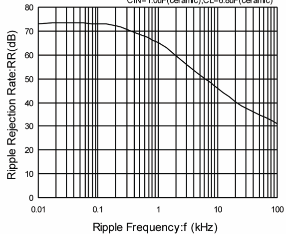
XC6210 (VOUT:5.0V)
