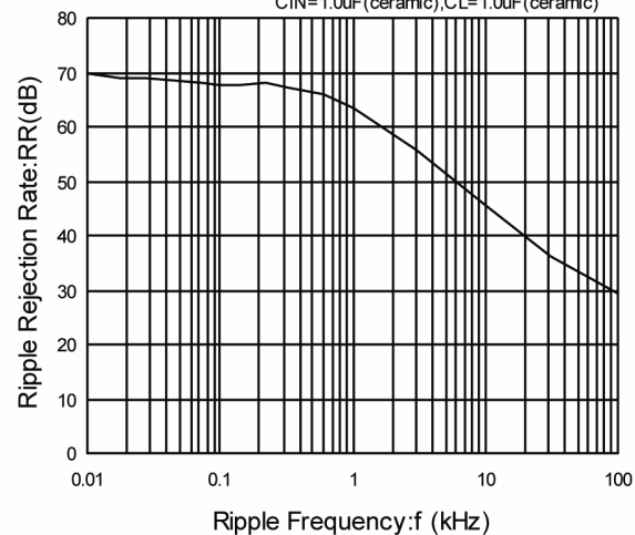
XC6210 (VOUT:5.0V)
