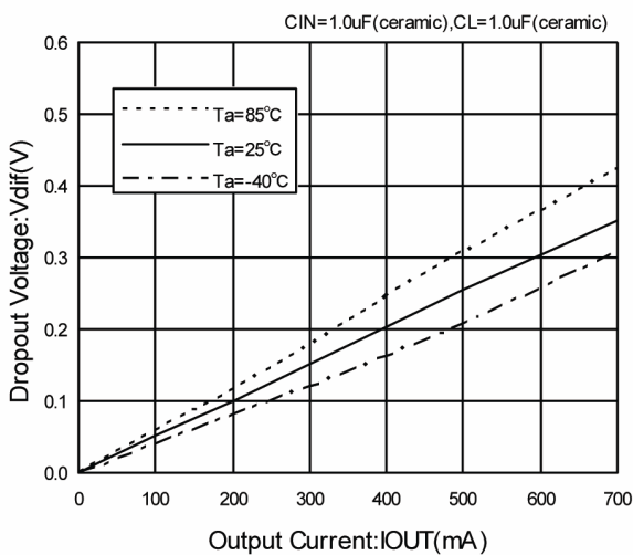
XC6210 (VOUT:3.0V)
