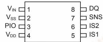
DS2751E 8-Pin TSSOP Package
