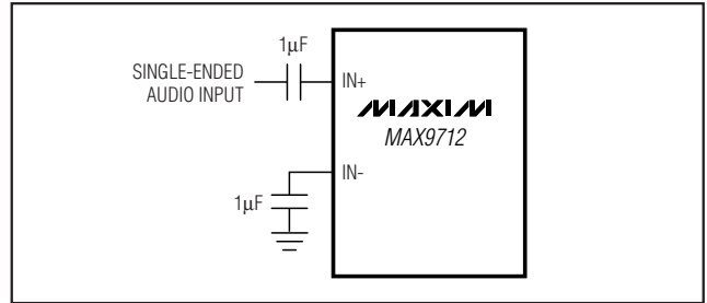
图 6. 单端输入
