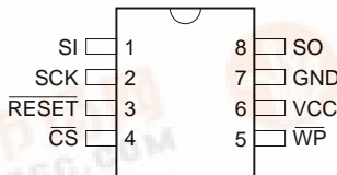
SOIC
