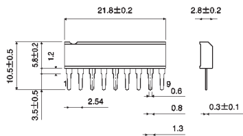
SIP9
