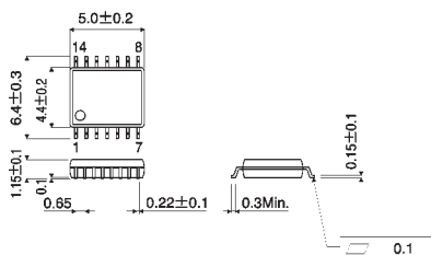
BA3308FV
