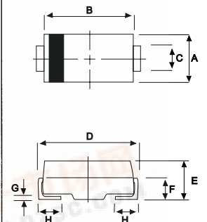
DO-214AC(SMA)
