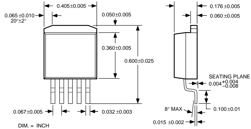
TO-263-5 (U)
