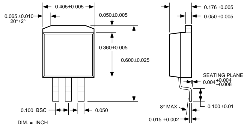
TO-263-3 (U)
