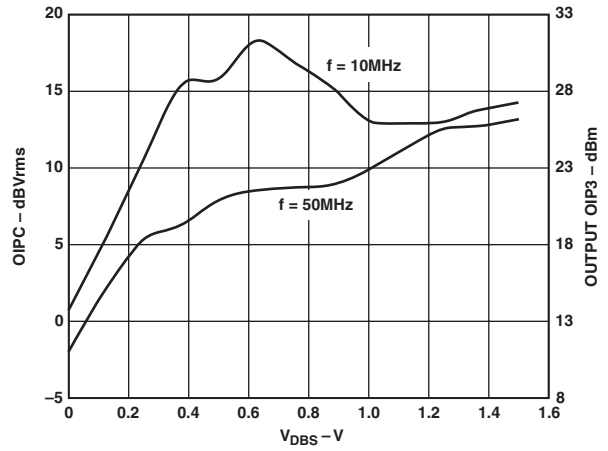
TPC 28. Output IP3 vs. V_{DBS}
