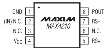
μMAX
