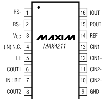
TSSOP
