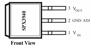
TO-263Package
