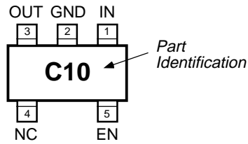
SOT-23-5 (M5)
