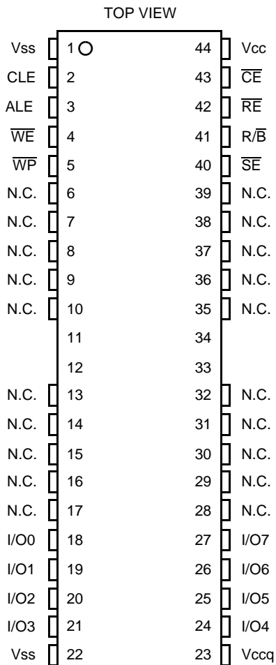
FPT-44P-M07
