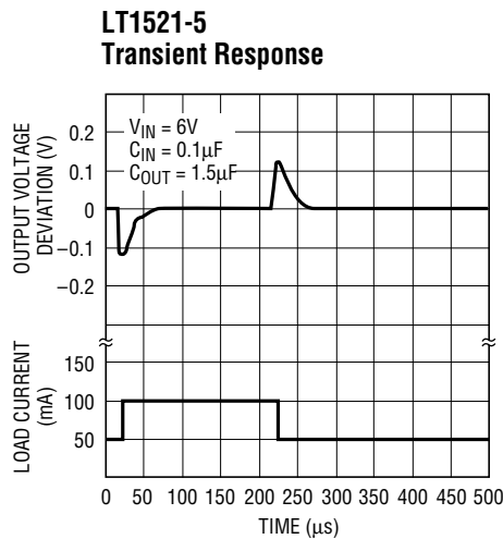
LT1521 • TPC33
