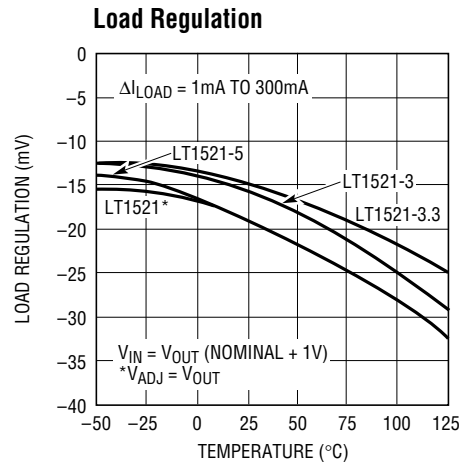
LT1521 • TPC32
