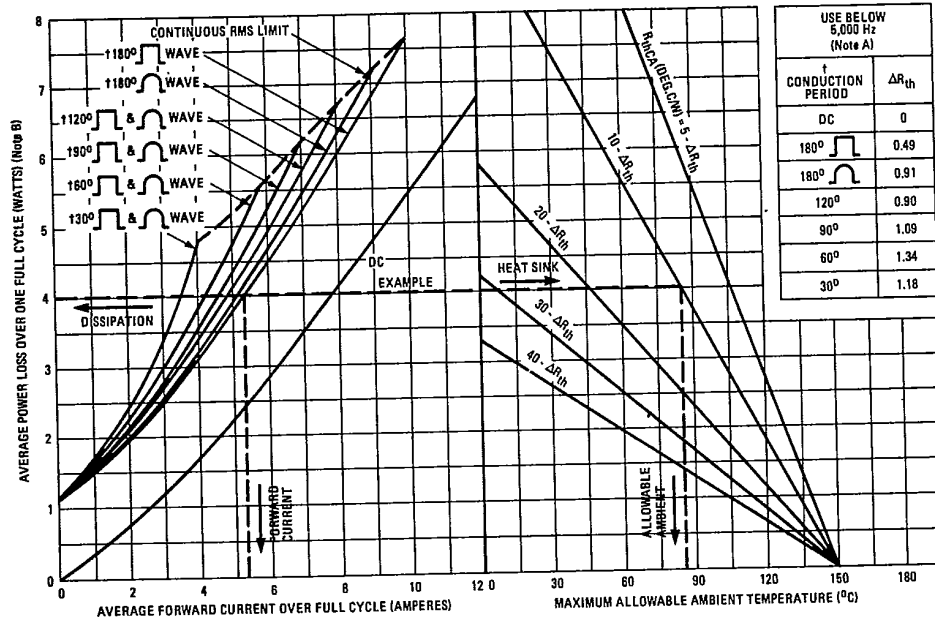
Fig. 9 - Thermal Nomogram
