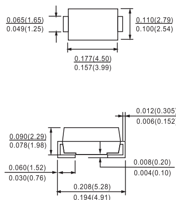
DO-214AC(SMA)
