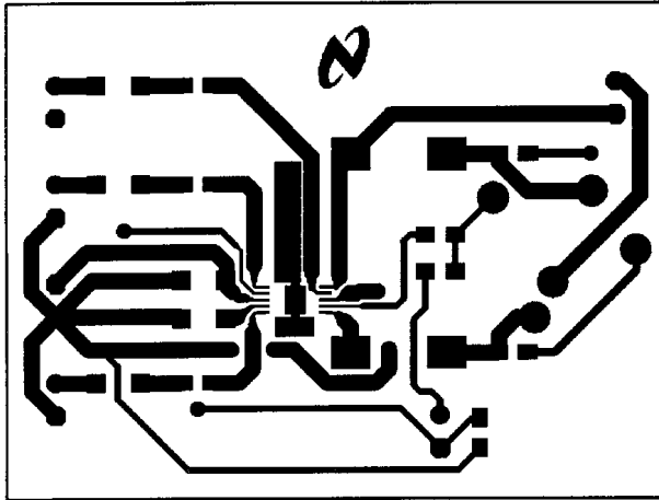
Top Layer
