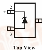
SOT-23-3 (M)
