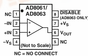
SOIC-8 (R)
