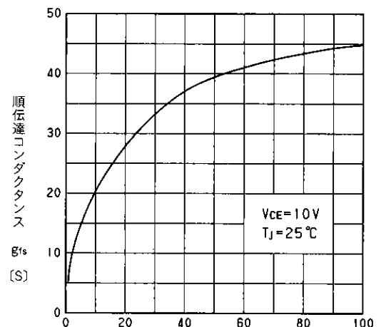
順伝達コンダクタンス-コレクタ電流特性(標準値) Typical Transconductances
