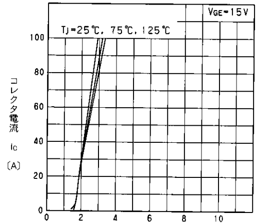
飽和電圧-コレクタ電流特性(標準値) V_{CE(sat)}-I_c Characteristics
