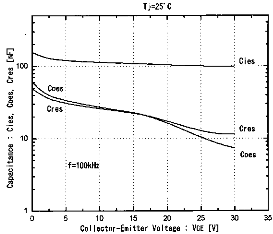
容量—コレクタ・エミッタ間電圧特性
