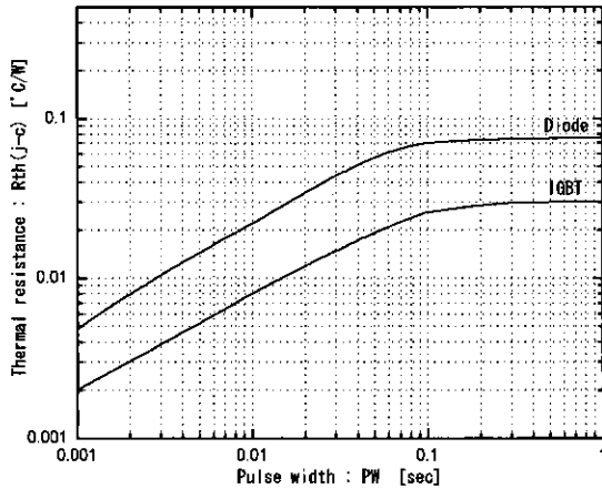
過渡熱抵抗特性
