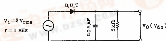
Fig. : TEST CIRCUIT
