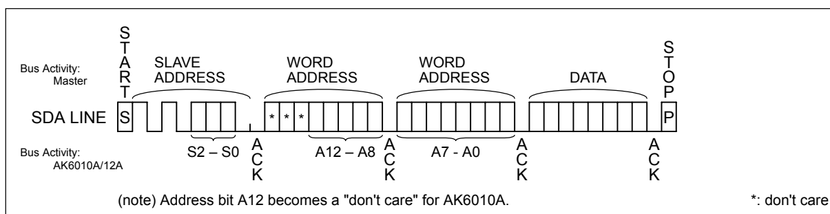
BYTE WRITE
