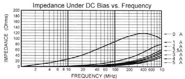
MLB-201209-0090PU
