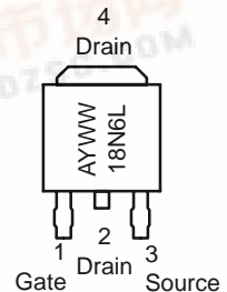
DPAK CASE 369C STYLE 2
