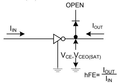
2. V_{CEO(SAT)}, hFE
