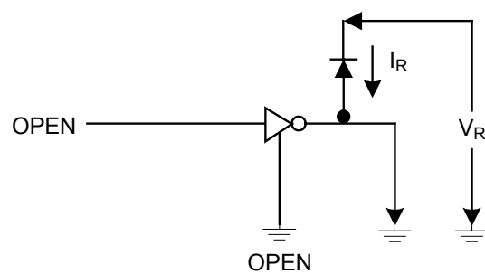
6. I_R
