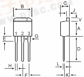
TO-262 (I 2 -PAK)
