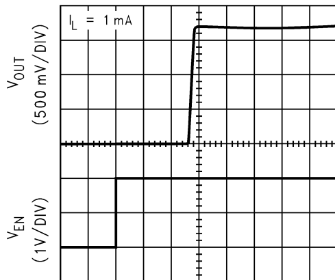
TIME (50 \mu s /DIV)
