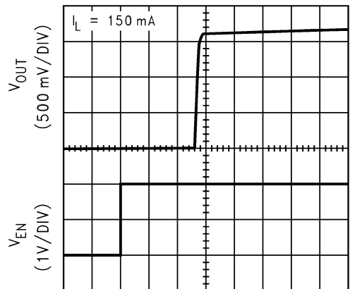
TIME (50 \mu s /DIV)
