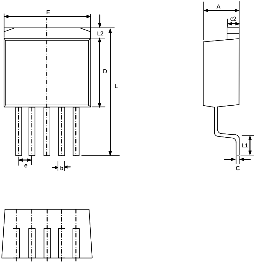
TO-263-5 Package
