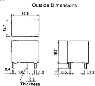
TX1
