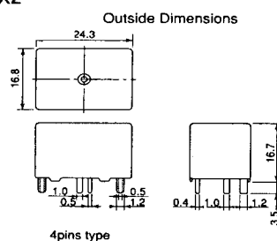
TX2
