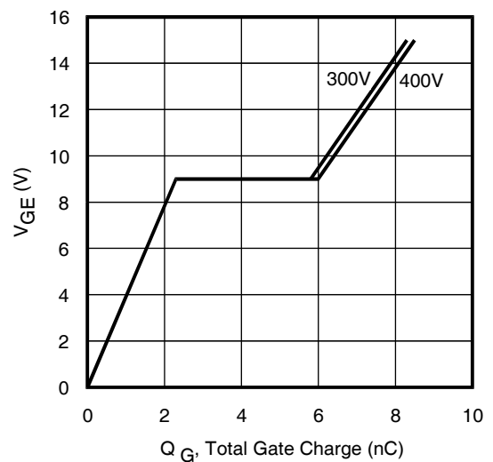
Fig. 24 - Typ. V_{GE} vs. Q_G
