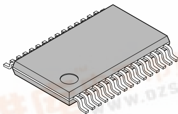
(FPT-30P-M04)
