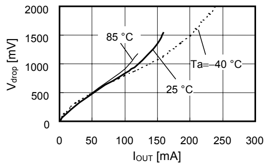
S-818A50A
