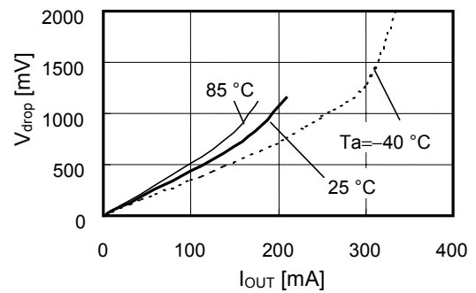
S-818A30A
