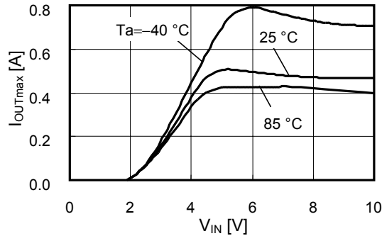
S-818A50A
