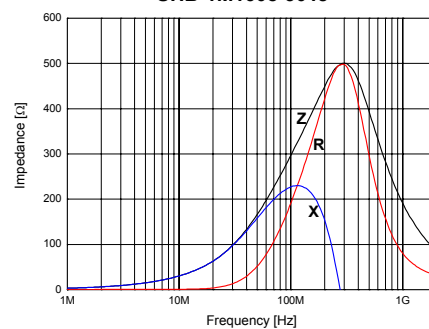
SHB-1M1608-301J
