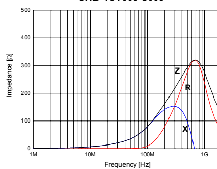
SHB-1S1608-800J
