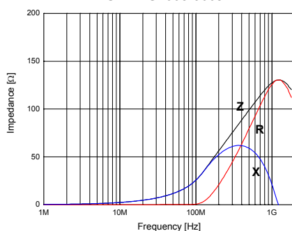
SHB-1S1608-300J
