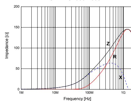
SHB-1S1608-400J
