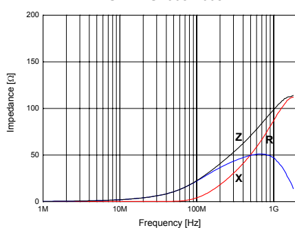
SHB-1S1608-200J
