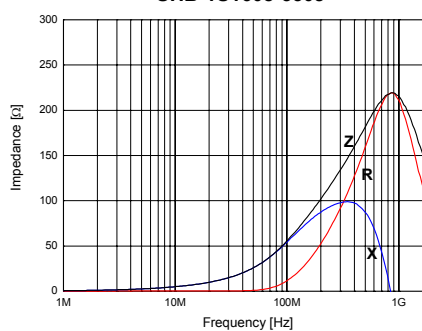
SHB-1S1608-550J
