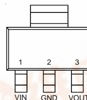
SOT-223
