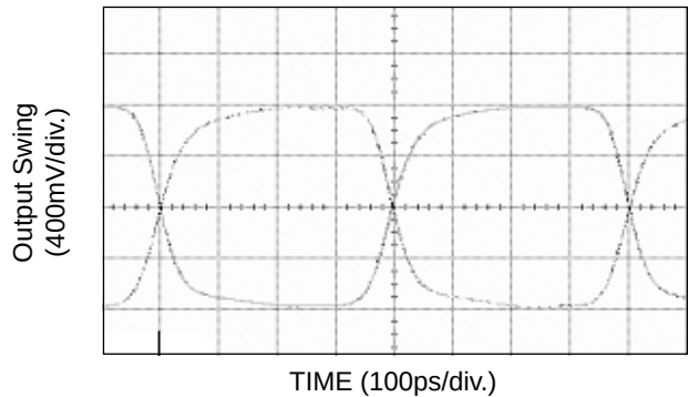
1.25GHz Output (Q – I/Q)
