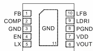
VDFN-10L 3x3
