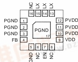
WQFN-16L 3x3
