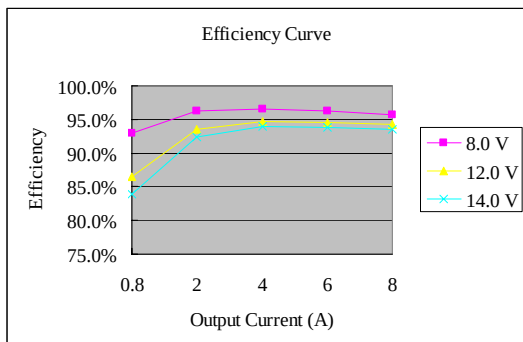
Vo=5.0 V
