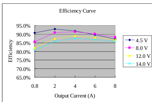
Vo=1.5 V
