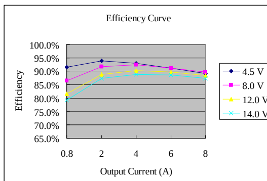
Vo=1.8 V
