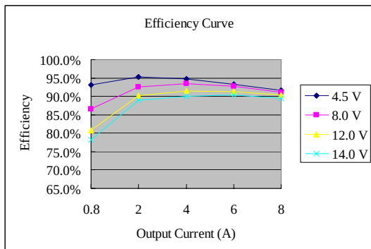
Vo=2.5 V
