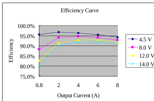
Vo=3.3 V
