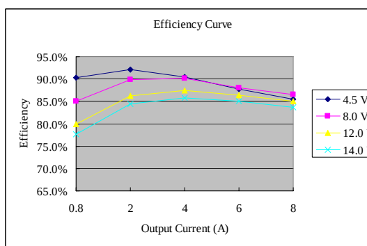
Vo=1.2 V
