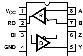
ISL3170E, ISL3173E, ISL3176E (SOIC) TOP VIEW
