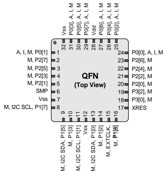
CY7C60333-LFXC Device
