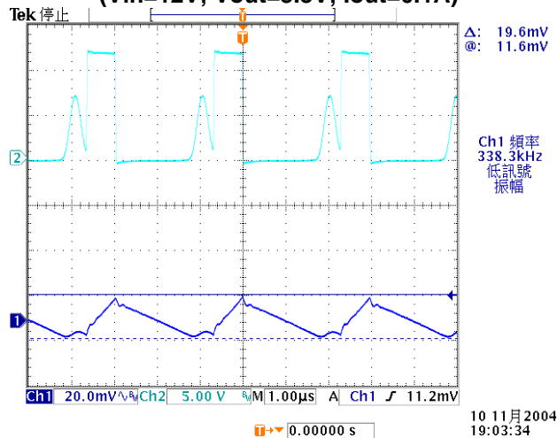
AP1510 Vout Ripple (Vin=12V; Vout=3.3V; Iout=0.1A)
