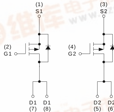
P-Channel MOSFET
