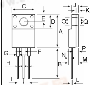
ITO-220AB
