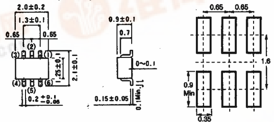
UMX11N (UMT6)
