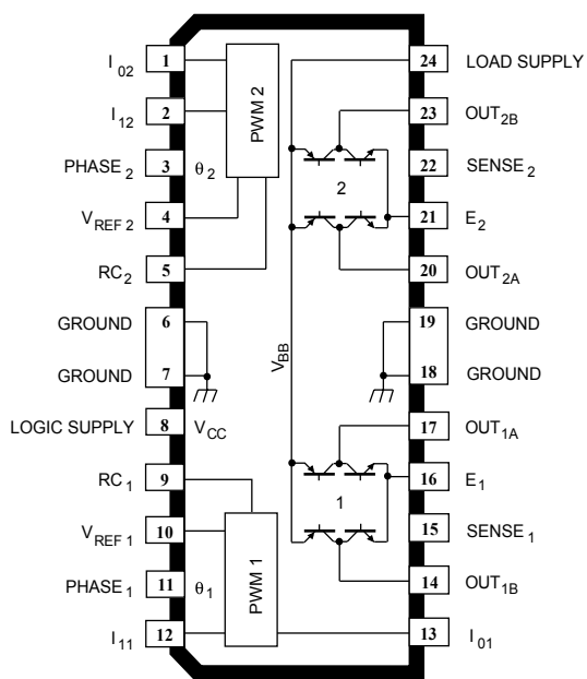
UDN2916LB (SOIC)
