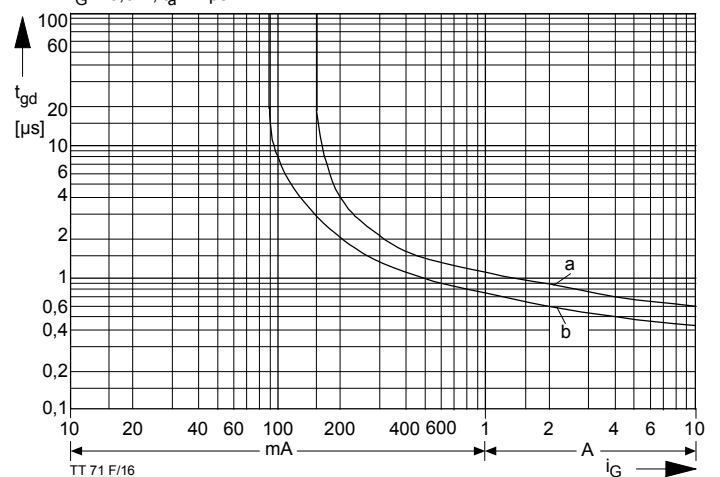
TT 71 F/16 Bild / Fig. 16 Zündverzögerung/Gate controlled delay time t_{gd} , DIN 41787, t_a = 1 \mu s, t_{vj} = 25^\circ C . a - äußerster Verlauf/limiting characteristic b - typischer Verlauf/typical characteristic
