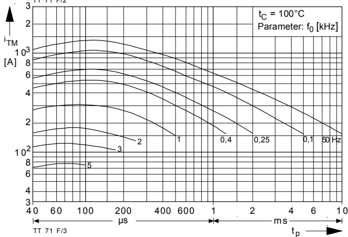
Bild / Fig. 1, 2, 3 Höchstzulässige Strombelastbarkeit in Abhängigkeit von der Halbschwingungsdauer für einen Zweig bei: sinusförmigem Stromverlauf, der angegebenen Gehäusetemperatur t_c , Vorwärts-Sperrspannung v_{DM} \leq 0,67 V_{DRM} , Freierzeitzeit t_0 gemäß 5. Kennbuchstaben, Spannungssteilheit dv_T/dt gemäß 6. Kennbuchstaben.
