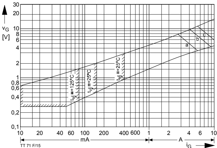
TT 71 F/15 Bild / Fig. 15 Steuercharakteristik mit Zündbereichen / Gate characteristic with triggering areas, v_G = f(i_G), v_D = 6 V
