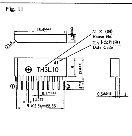
外形図 Outline Dimensions
